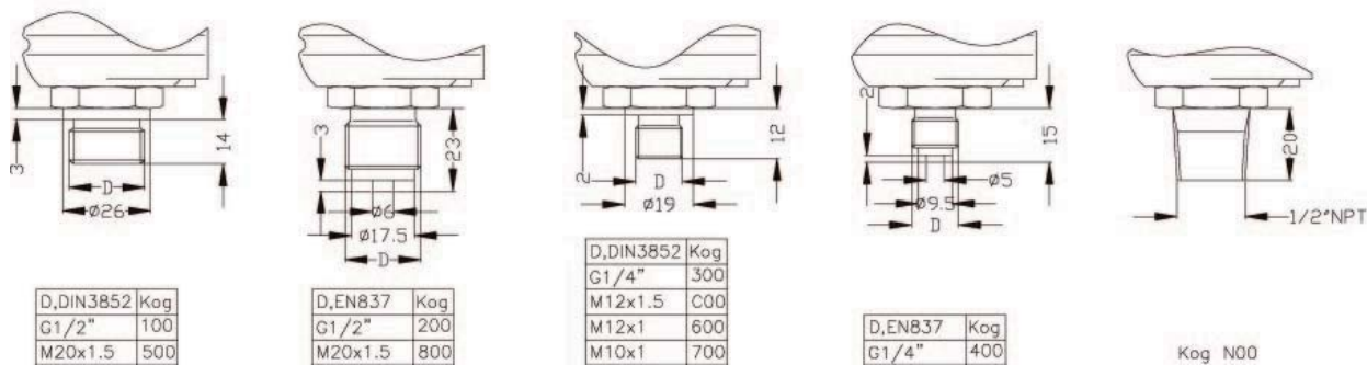
Рисунок Б.2 – Датчик НМР 331 с разделителем сред (верхний предел измерения не более 4 МПа).
